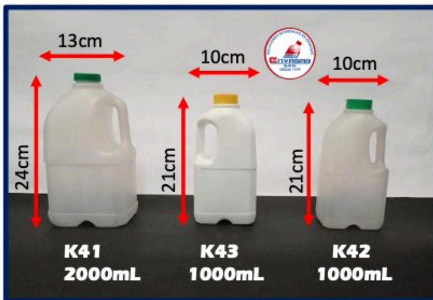
Envases lácteos Material: PE – Color Cuerpo Natural y Blanco, Tapa Variados
