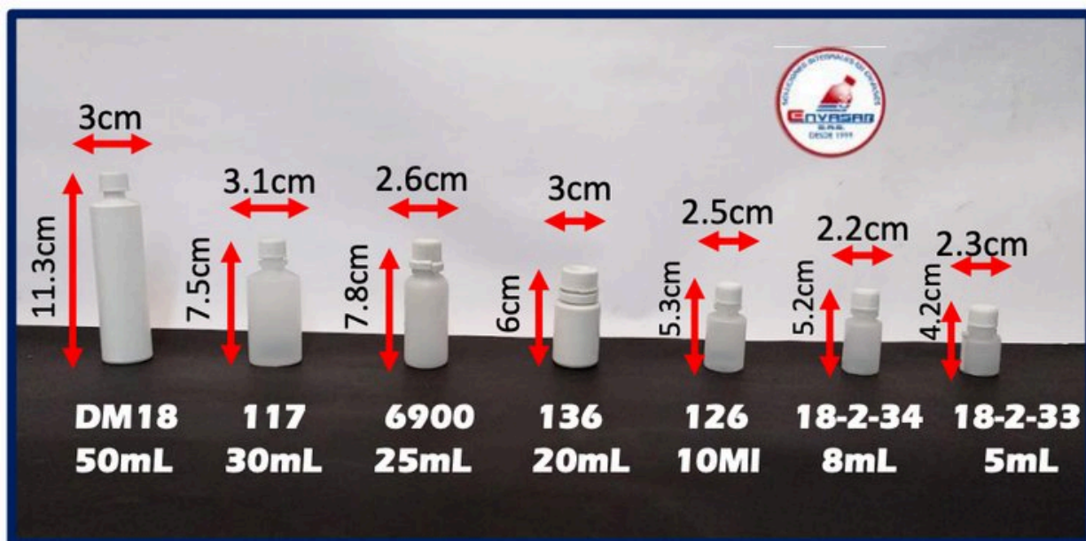
Envases farmacéuticos Material: PE – Color Blanco y Natural
