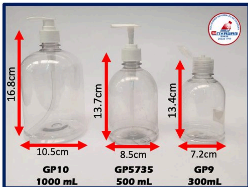
Envases Campana con tapa o válvula dosificadora Material: PET – Boca 28mm – Color Transparente
