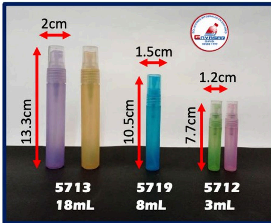
Envases Perfumeros Material: PP – Color Variados
