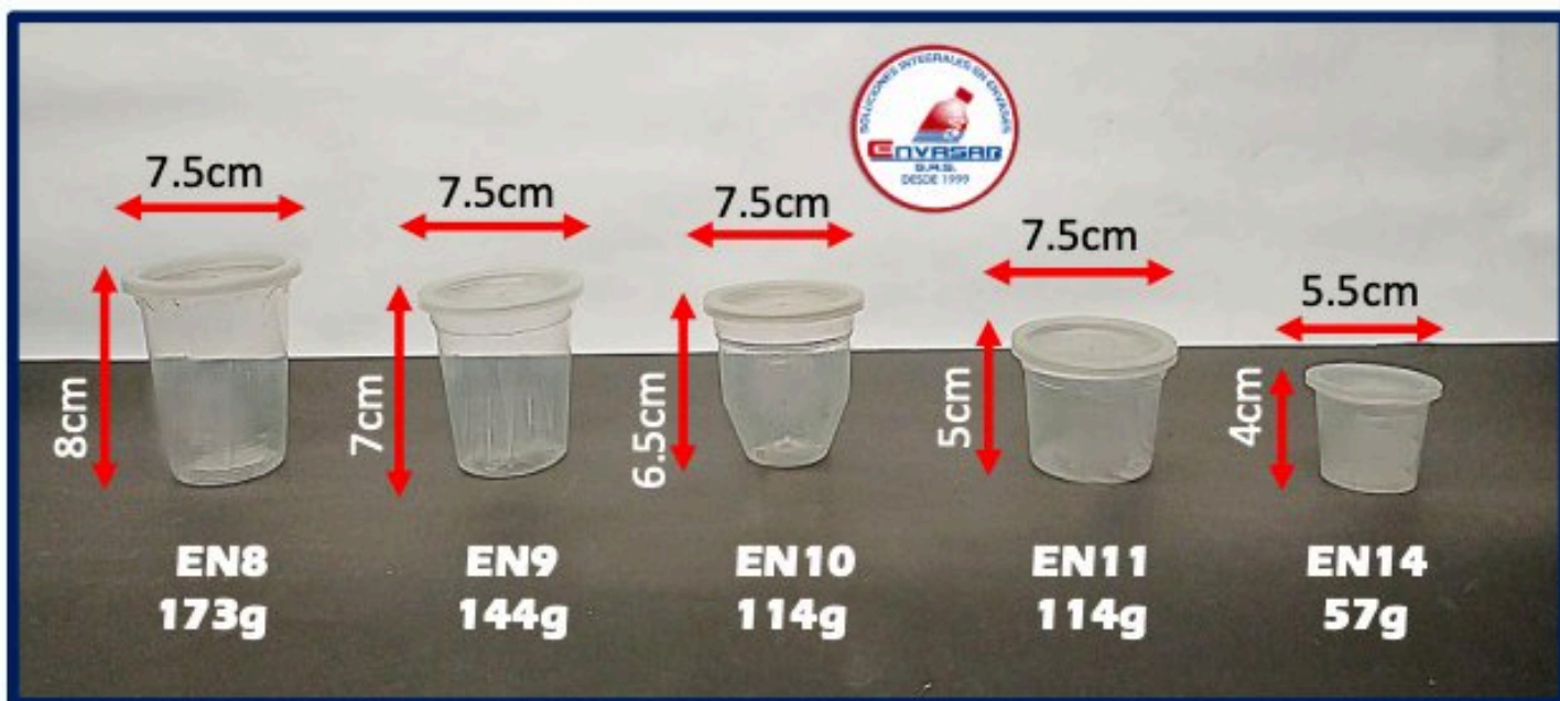
Envases para postres Material: PP – Color Natural
