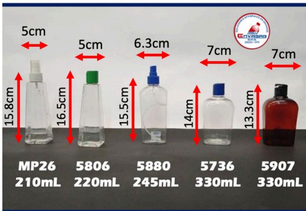
Envases cosméticos multiuso Material: PET – Color Transparente
