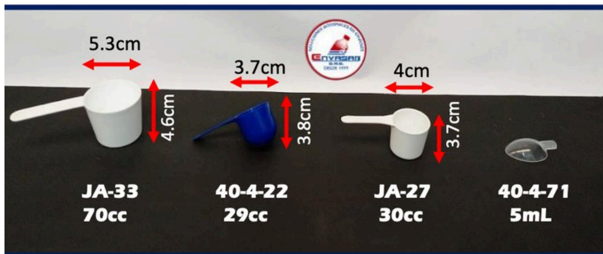
Cucharas dosificadoras Material: PP y PS – Color Variados
