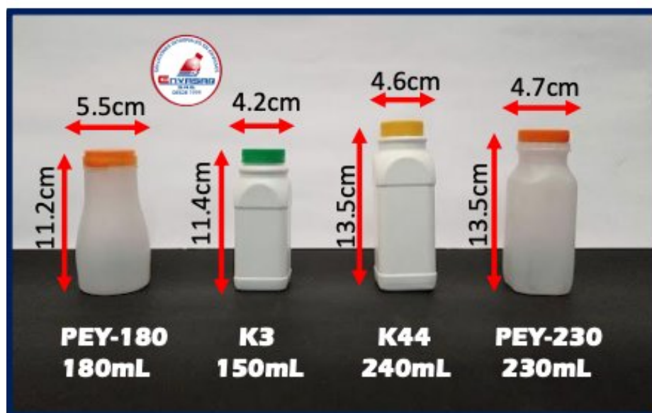
Envases lácteos Material: PE – Color Cuerpo Natural y Blanco, Tapa Variados
