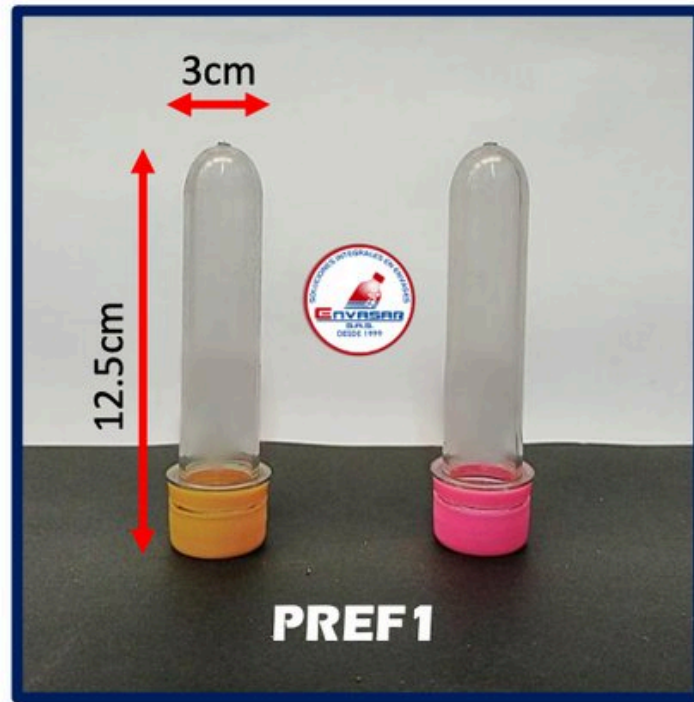
Preformas Material: PET – Color Transparente
