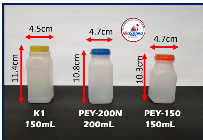
Envases lácteos Material: PE – Color Cuerpo Natural, Tapa Variados
