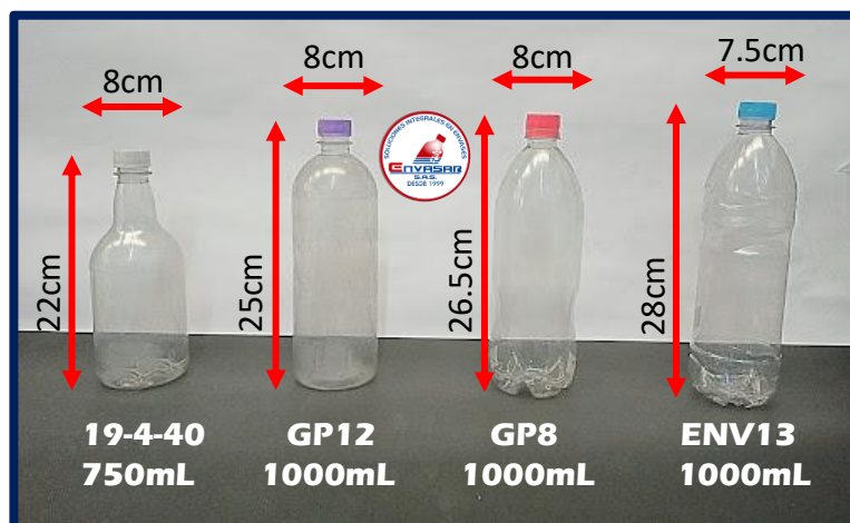
Envases para liquido Material: PET – Color Cuerpo Transparente, Tapa Variados
