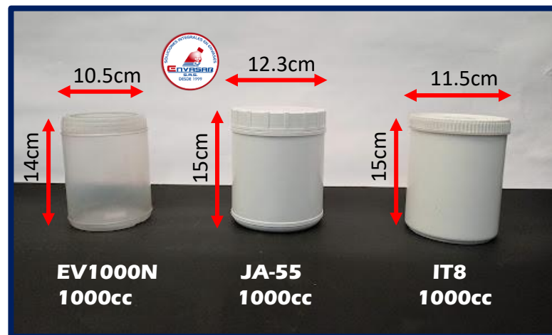
Envases nutricionales Material: PP y PE – Color Natural y Blanco
