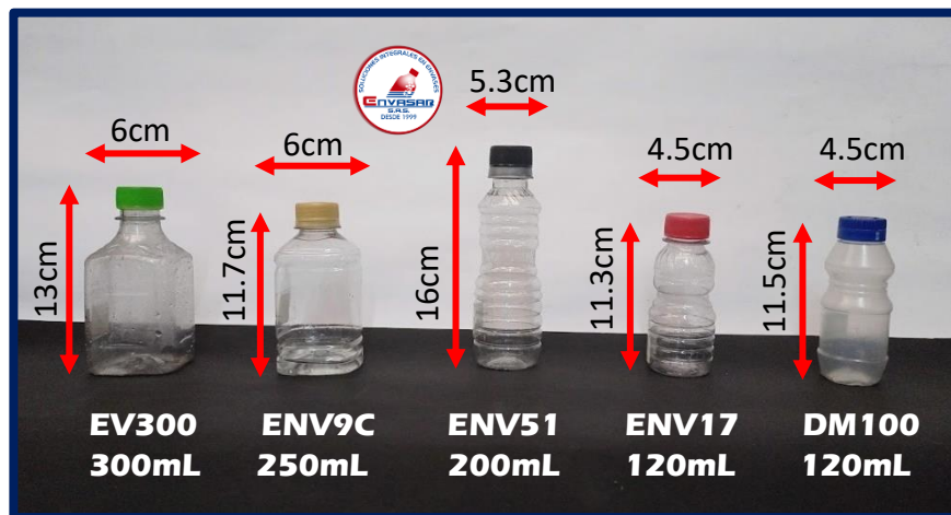
Envases para liquido Material: PET y PP – Color Cuerpo Transparente y Natural, Tapa Variados
