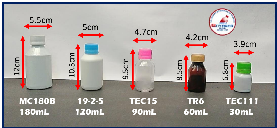
Envases jaraberos Material: PET - Boca 28mm - Color Blanco, Cristal y Ámbar
